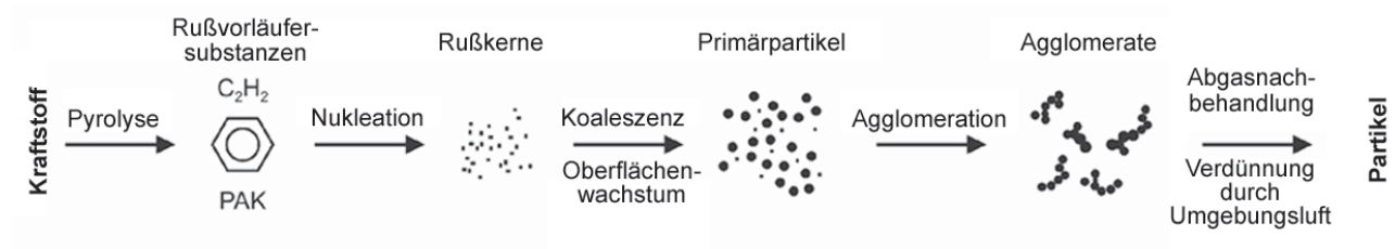
Abb. 5-8: Partikelbildung vom Kraftstoff bis zum verdünnten Abgas (nach Tree und Svensen, 2007; nach Schaak 2012)
